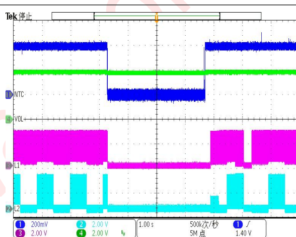
充电状态: NTC-10K 动作波形图, 5VIN@3.8VBAT
