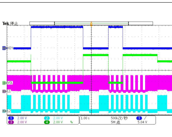
充电状态: ENH↔ENL 动作波形图, 5VIN@3.8VBAT
