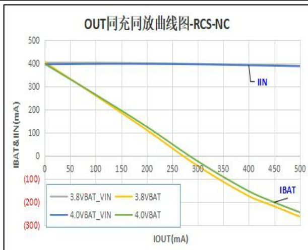
充电和放电状态波形图:
