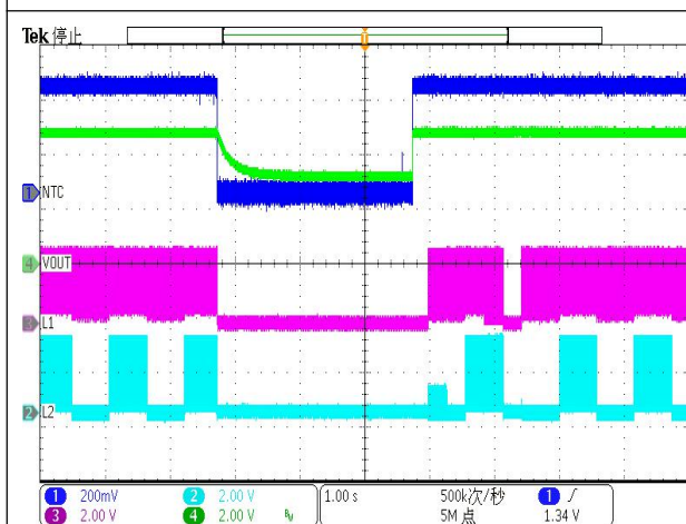
充电状态: NTC-10K 动作波形图, 5VIN@3.8VBAT
