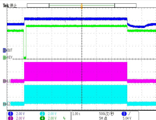
待机模式：单击 KEY 键波形图，4.2VBAT
