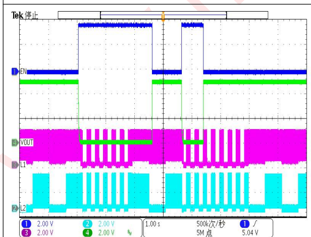
充电状态: ENH↔ENL 动作波形图, 5VIN@3.8VBAT
