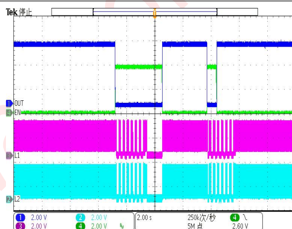
放电过程中：ENH↔ENL 动作波形图，3.8VBAT
