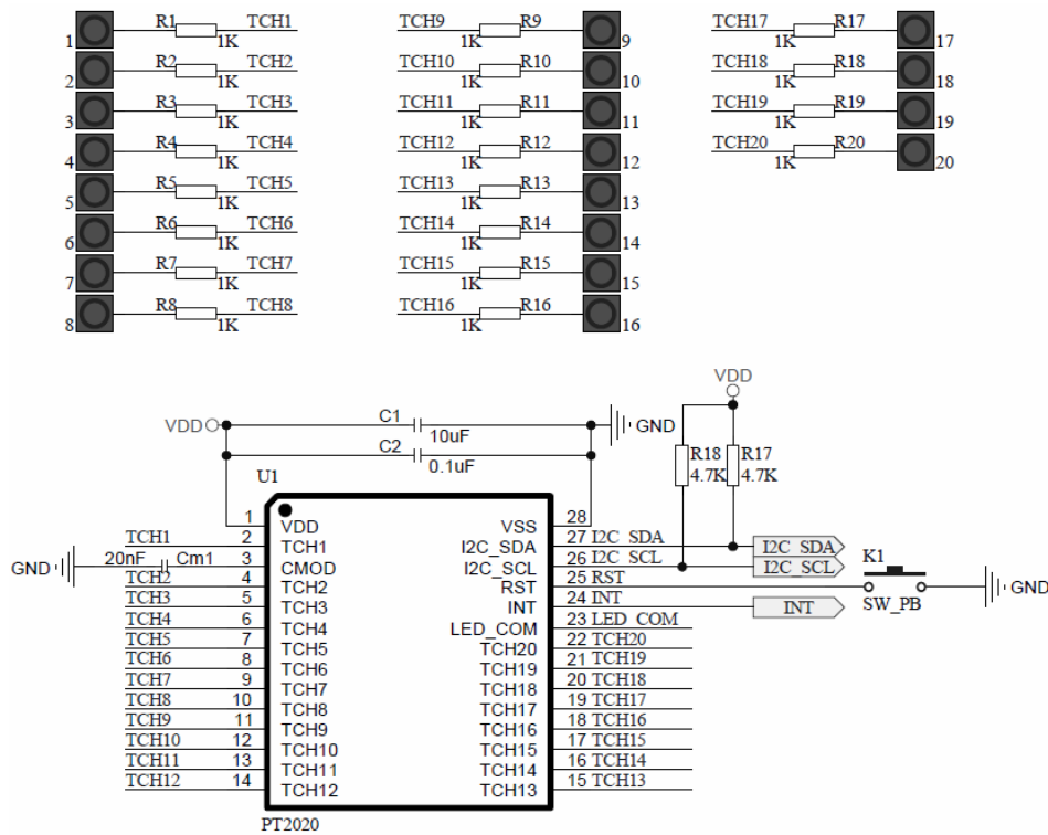
图 3 典型应用电路
