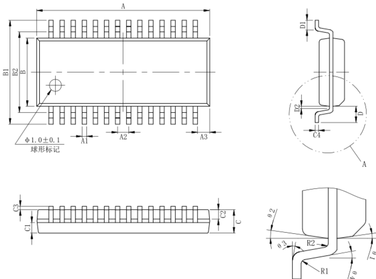
图 5 SSOP28 封装图
