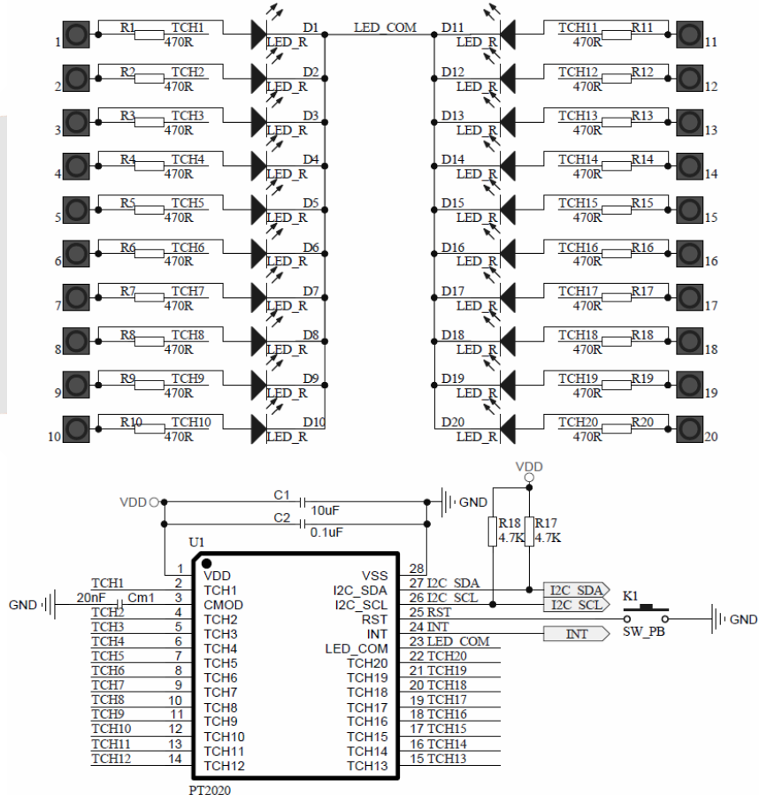
图 4 触摸复用 LED 驱动典型应用电路
