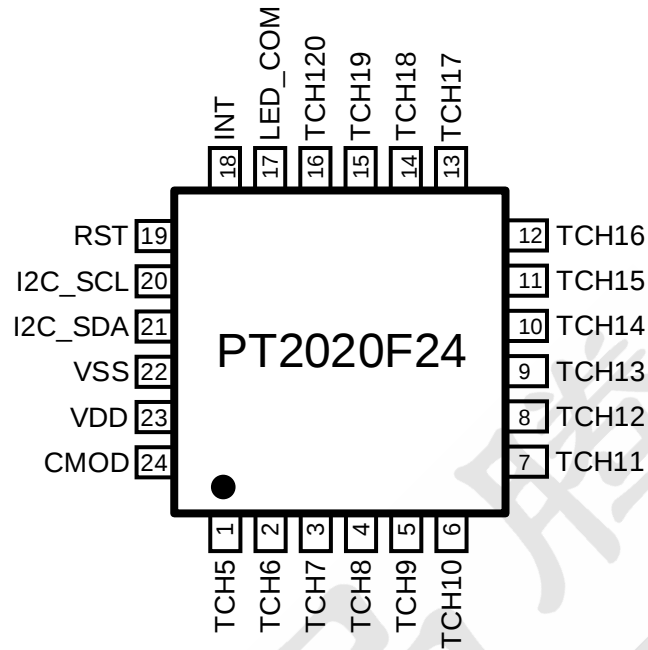
图 1 管脚示意
