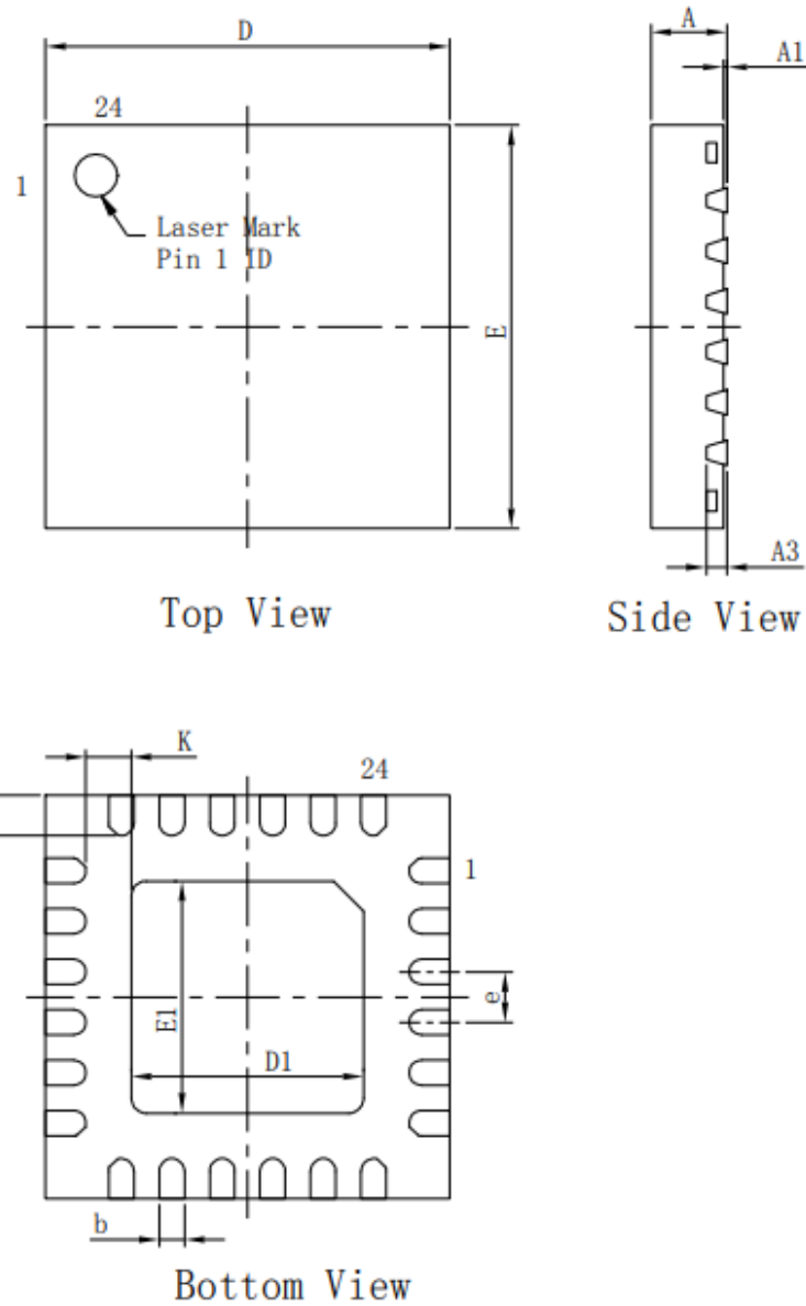
图 6 QFN24 封装图
