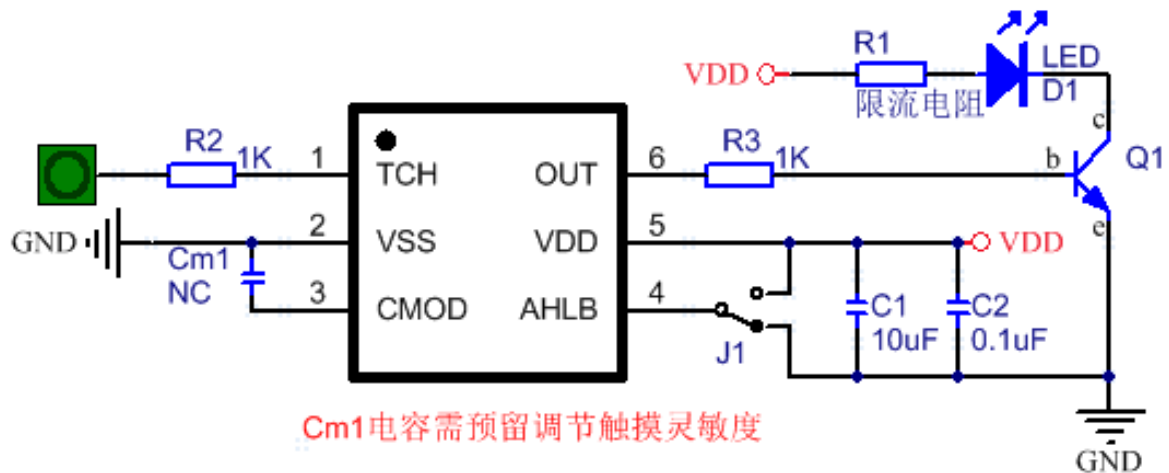
图 2 标准应用电路
